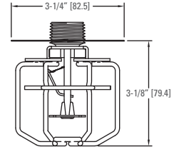
Proteção e Shield com sprinkler mod GL 112 Pendente 3/4"
