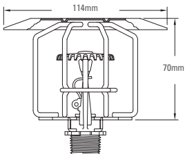
Proteção com sprinkler mod G - Upright
