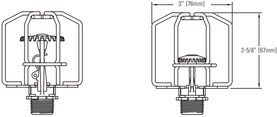
Proteção com sprinkler mod G - Upright
