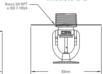
Shield com sprinkler mod F1FR LO
