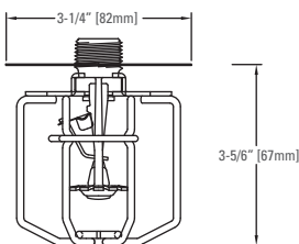
Proteção e Shield com GRF - Pendente Nível intermediário 1/2"
