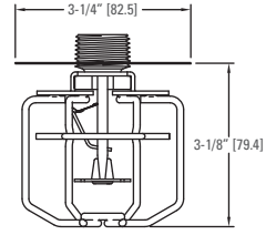
Proteção e Shield com sprinkler mod GL 112 Pendente 3/4"
