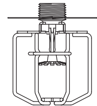
Proteção e Shield com sprinkler mod F1 - Pendente Nível intermediário 3/4"
