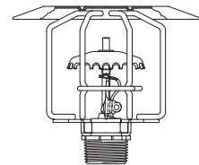
Proteção e Shield com sprinkler mod G XL0231 3/4" Upright - Nível intermediário
