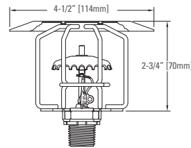
Proteção e Shield com sprinkler mod G XL0231 1/2" Upright - Nível intermediário
