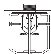
Proteção e Shield com sprinkler mod F1
