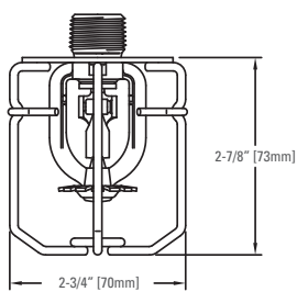
Proteção com sprinkler mod G Pendente
