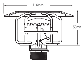
Proteção e Shield com sprinkler mod GL 112 Upright 1/2"
