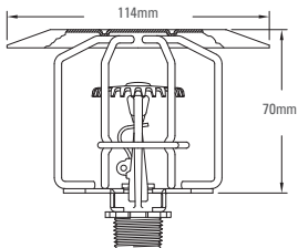
Proteção com sprinkler mod G - Upright
