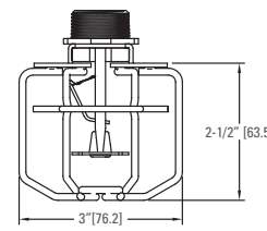
Proteção com sprinkler mod GL 112 Pendente 3/4"
