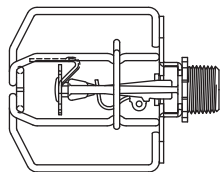
Proteção com sprinkler mod G - Horizontal
