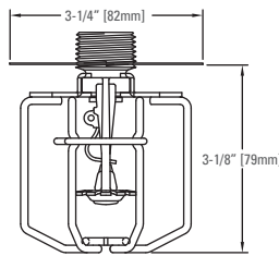
Proteção e Shield com sprinkler mod G - Pendente Nível intermediário 3/4"
