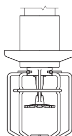
Proteção com sprinkler mod F3
