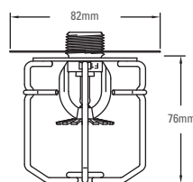
Proteção e Shield com sprinkler mod F1FR
