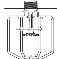
Proteção e Shield com F1 - Pendente Nível intermediário 1/2"
