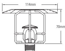
Proteção e Shield com sprinkler mod F1FR
