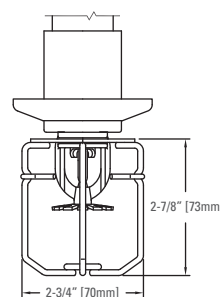
Proteção com sprinkler mod F3
