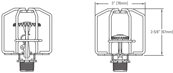
Proteção com sprinkler mod G - Upright
