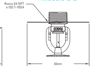
Shield com sprinkler mod F1FR LO
